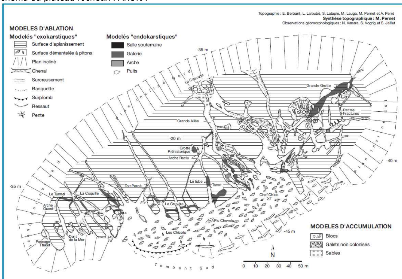
Figure 3 : Carte géomorphologique du massif d'Aroka. Geomorphologic map of the Aroka massif.
